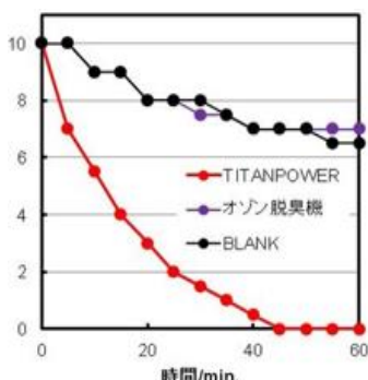
硫化水素
