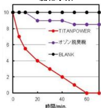
硫化水素
